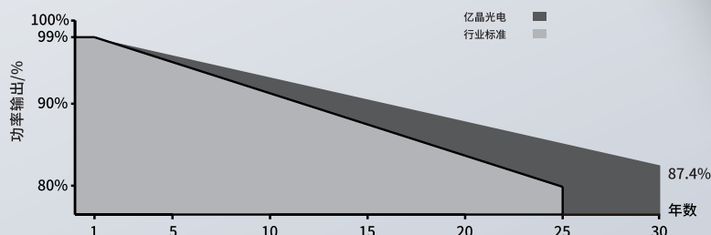
N型单晶组件线性功率保证
