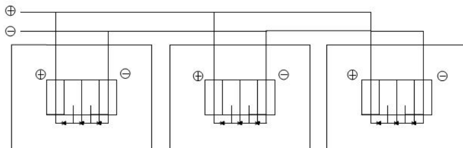
图 4 用于更大电流的串联
