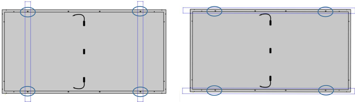
外四孔螺栓安装（横梁垂直于长边框）
