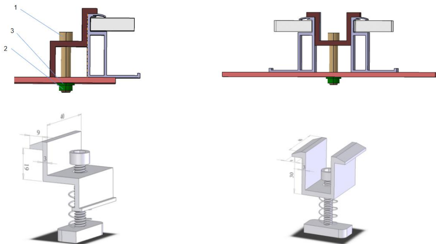
图 2 组件中间用夹具与组件边缘用夹具
