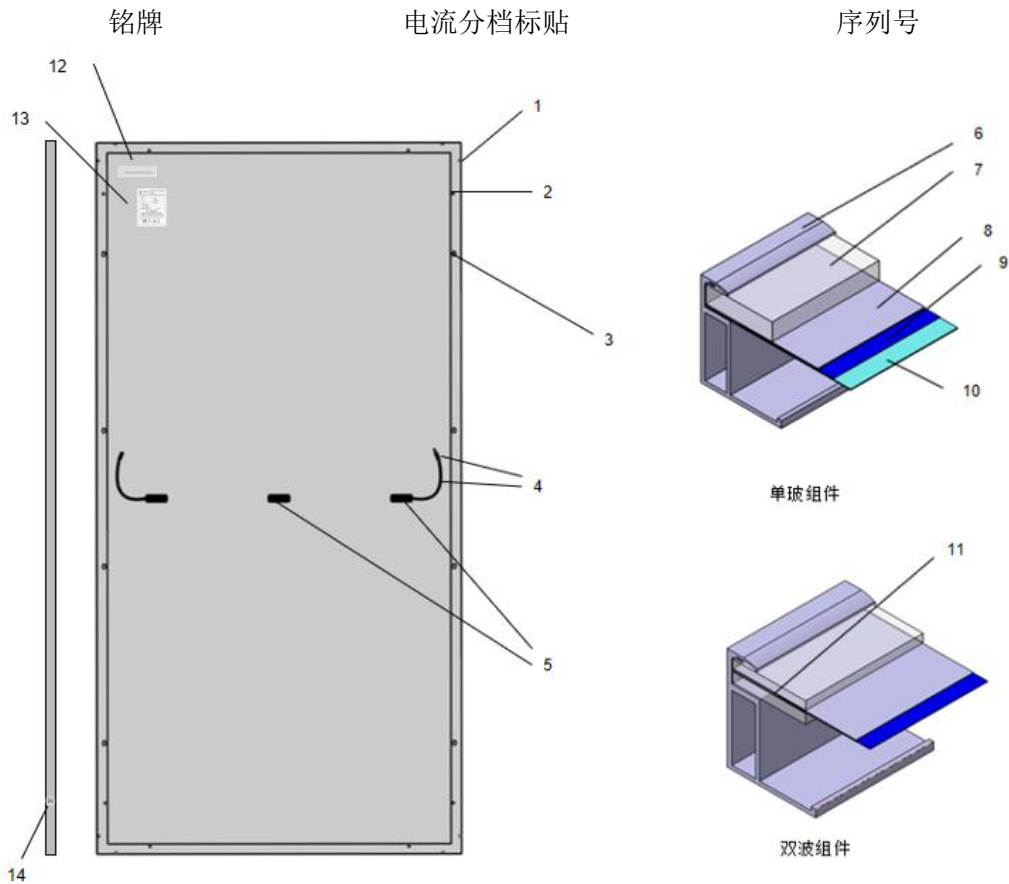
图 1 单面组件结构示意图和双面组件结构示意图
