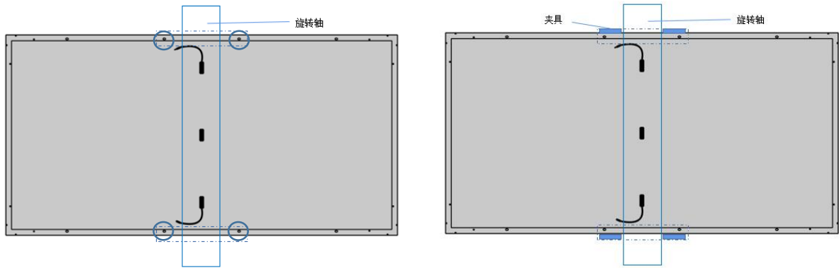
跟踪支架 1 排安装示意图：
