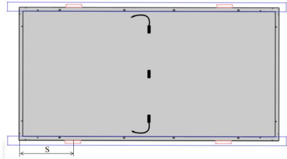
长边夹具安装 (横梁平行于长边框)
